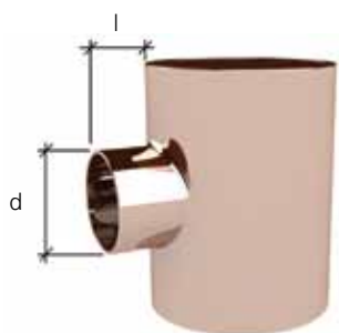
l \leq 1,5 \times d fig. 3.1.1
